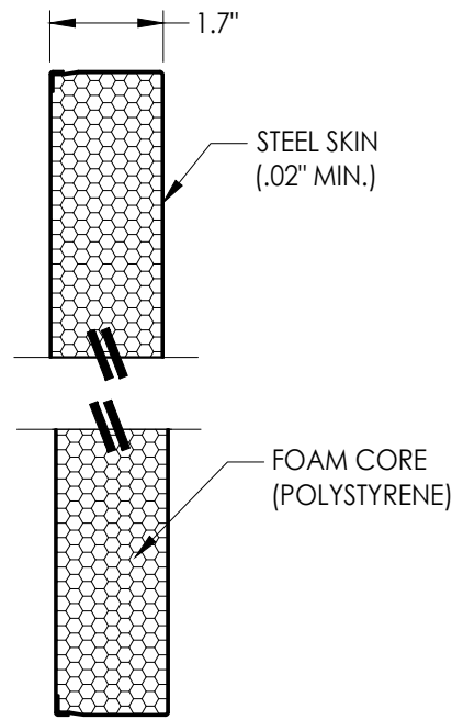
SECTION D-D
